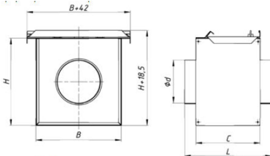
Габаритные размеры корпуса ФВ
