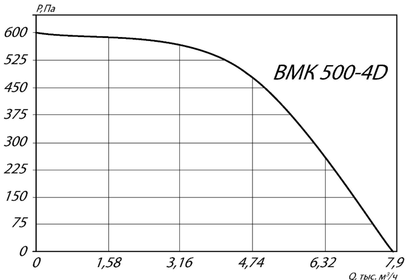
Аэродинамические характеристики крышного вентилятора ВМК 500
