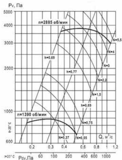
Аэродинамическая характеристика вентилятора BP 132-30 №4,5 (1 исполнение)
