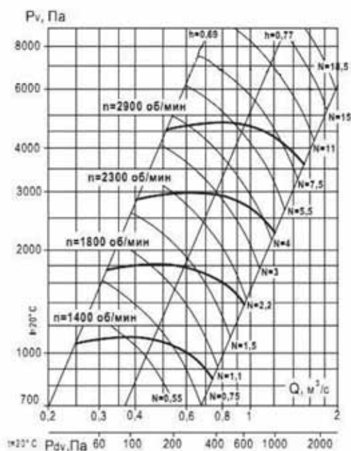
Аэродинамическая характеристика вентилятора BP 132-30 №5 (1 и 5 исполнение)
