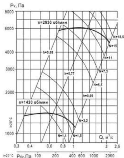
Аэродинамическая характеристика вентилятора BP 132-30 №5,6 (1 исполнение)
