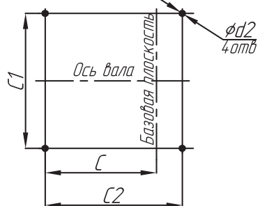
Схема расположения отверстий для крепления вентилятора ВР 132-30-4...10
