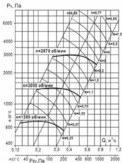
Аэродинамическая характеристика вентилятора BP 132-30 №4 (1 и 5 исполнение)
