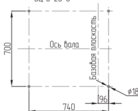
Схема расположения отверстий для крепления вентилятора ВЦ 6-20-8
